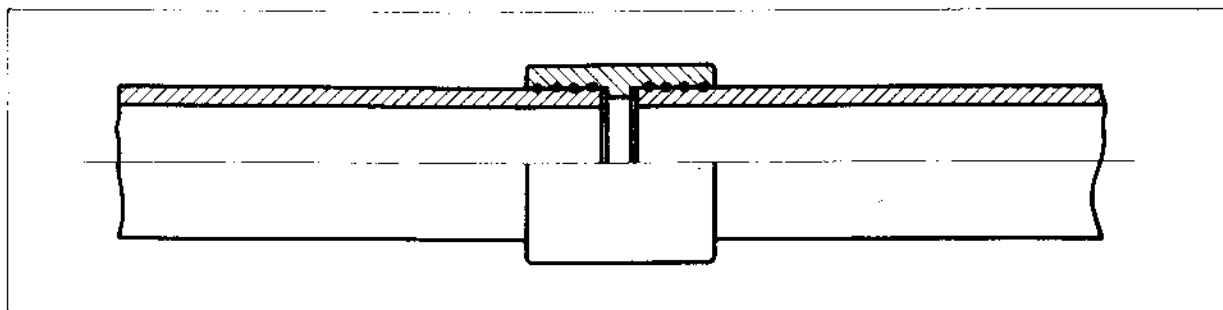
Fig. 2 - Manicotto di PE a.d. con elettroresistenza incorporata
