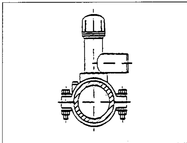
Fig. 29 - Collare di presa elettrosaldabile con T di derivazione.
