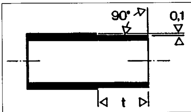
Fig. 16 - Raschiatura.
