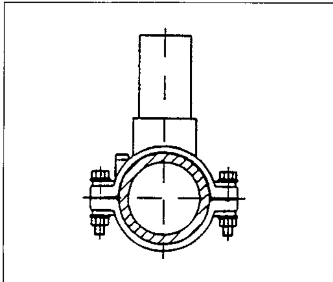
Fig. 27 - Collare di presa elettrosaldabile.
