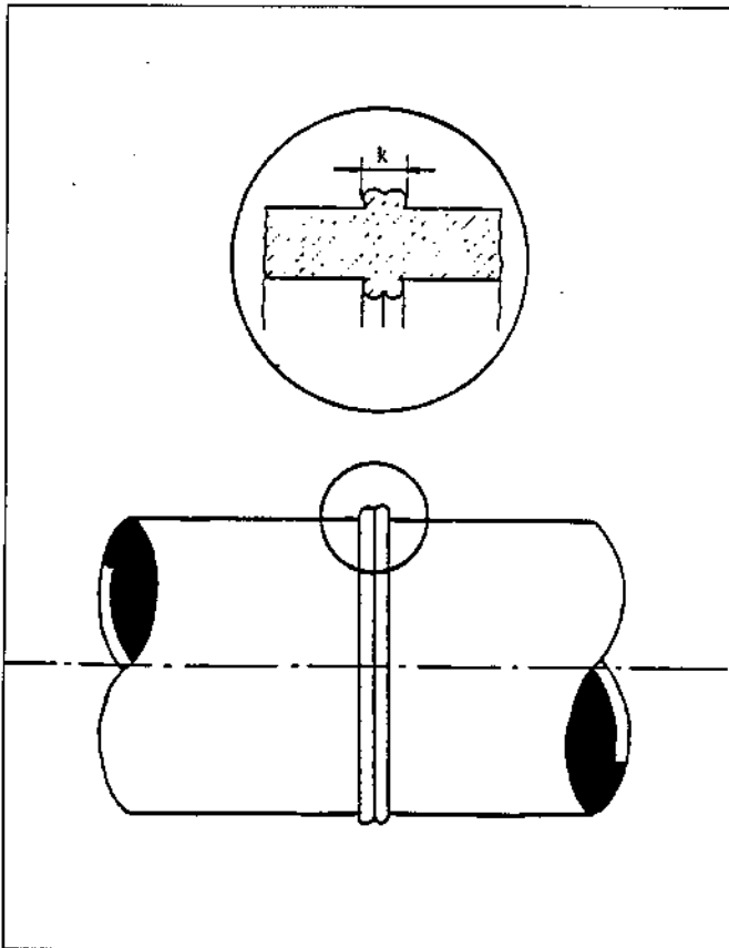
Fig. 25 - Cordolo della saldatura testa-testa.
