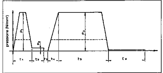
Fig. 20 - Diagramma saldatura testa-testa.
