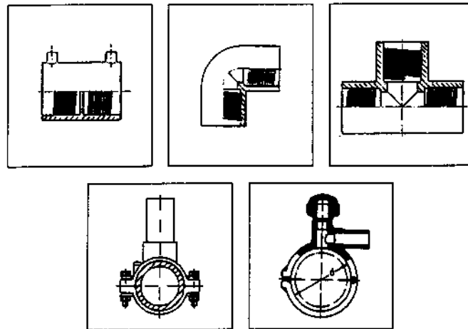
Fig. 2 - Elettrosaldabili.
