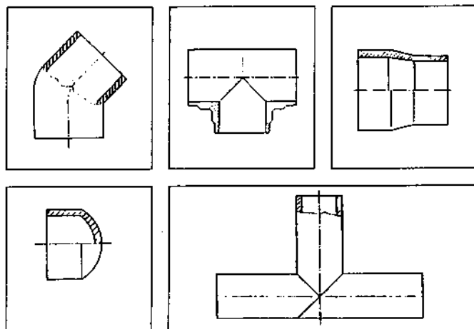
Fig. 1 - Pezzi speciali.
