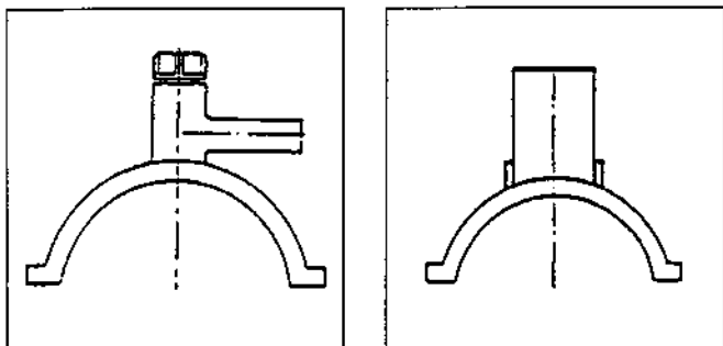
Fig. 28 - Selle elettrosaldabili.
