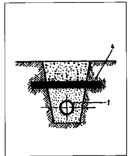
Fig. 7 - Protezione tubazione con piastra di cemento.
