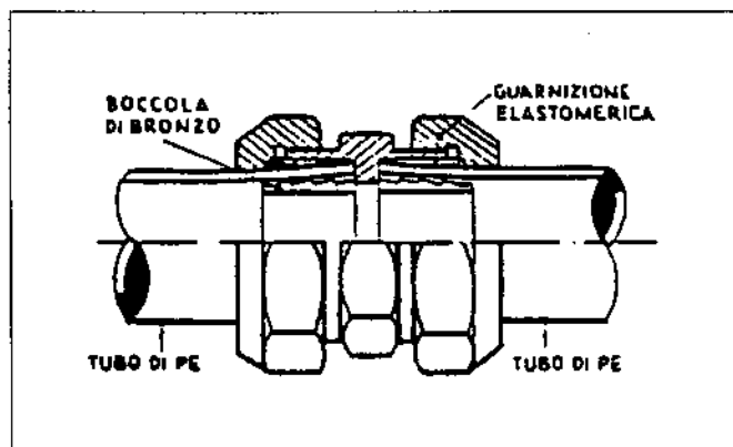
Fig. 30 - Giunto meccanico.
