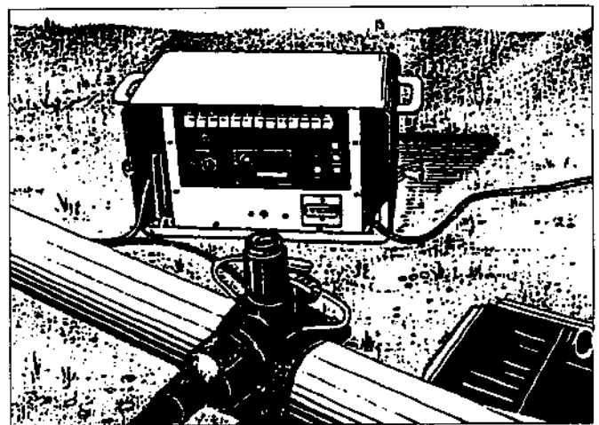
Fig. 15 - Saldatrice per elettrofusione.
