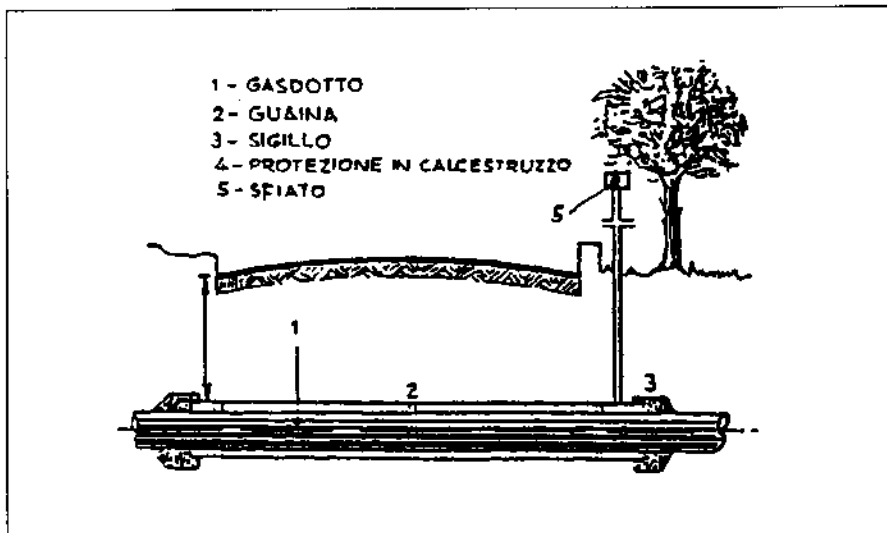
Fig. 6 - Interramento tubazione con guaina di protezione.
