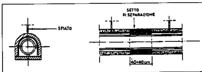
Fig. 8 - Tubazione in cunicolo.
