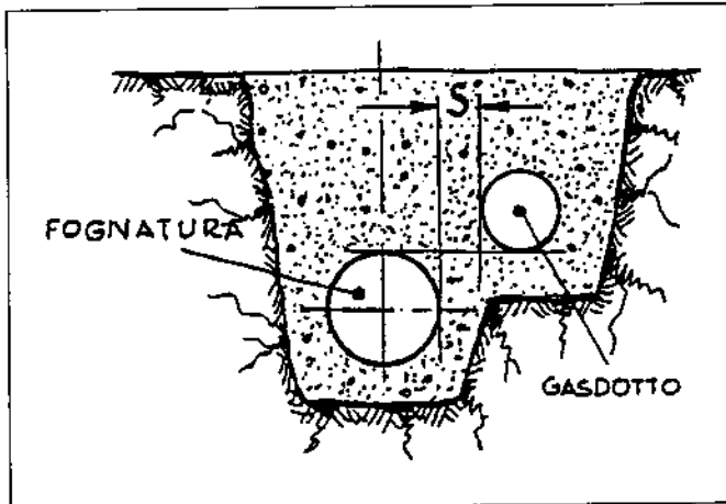
Fig. 9 - Parallelismo gasdotto-fognatura.
