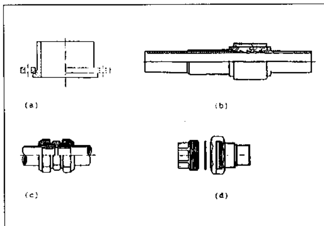
Fig. 3 - Giunti Pe/Fe.
