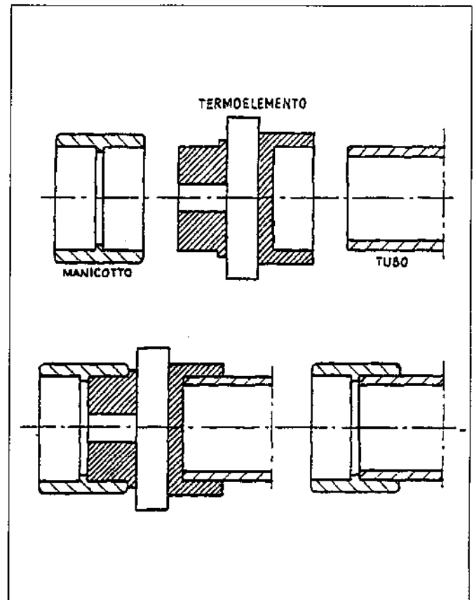
Fig. 26 - Saldatura per polifusione nel bicchiere.
