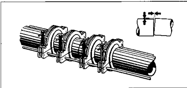
Fig. 19 - Controllo disassamento e complanarità.
